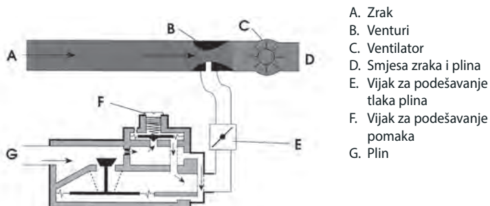
Skica A: funkcionalni dijagram
