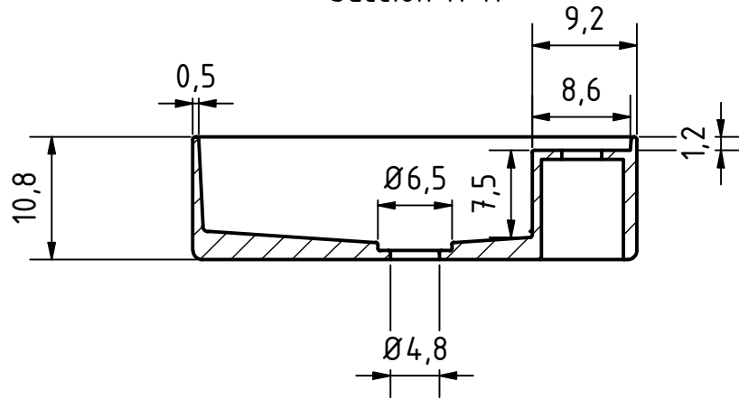
Sección H-H
